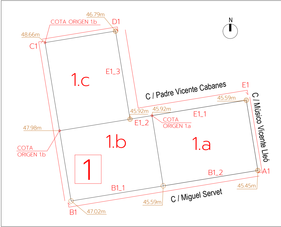
Planta de referencia (e: 1/700)
